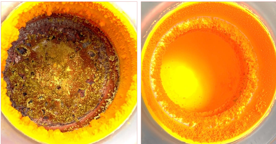
Fig III.4.5. Fin de la troisième sublimation, salammoniac off magnetite. Récipient de réaction du fond à gauche, tête sublimateur à droite.
