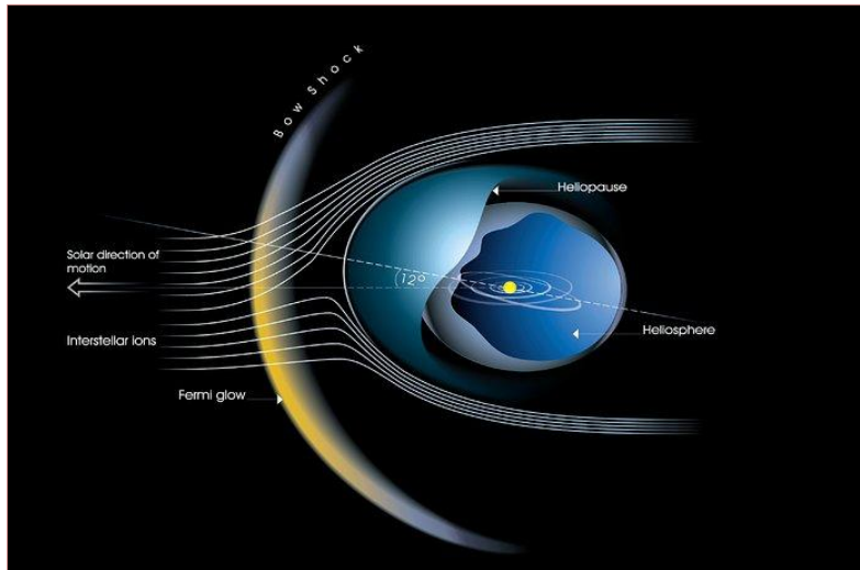
Fig 1.10.1. L'héliosphère et sa relation avec le vent interstellaire. https://esahubble.org/images/heic9911b/
