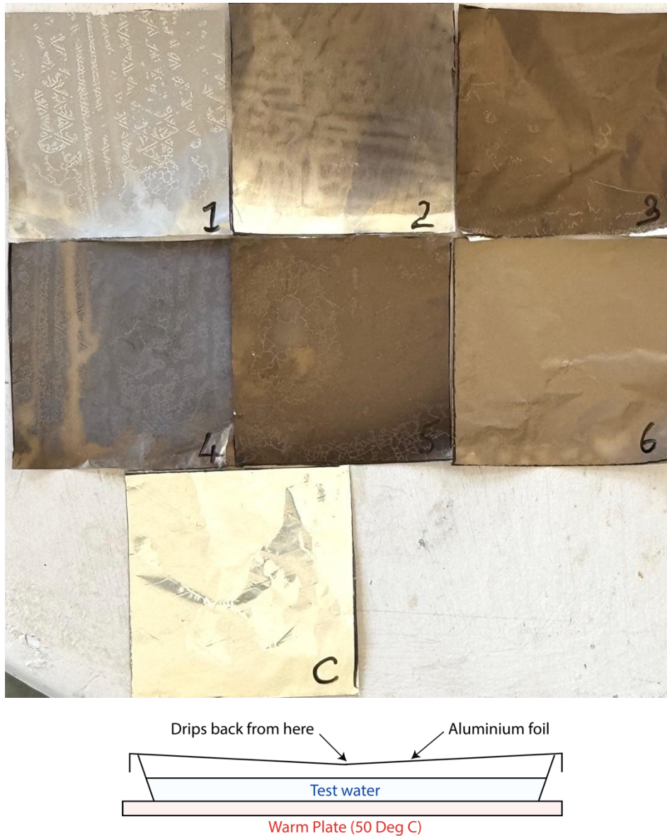
Fig 1.9.12. La dorure du papier d'aluminium par divers échantillons d'eau en légère vaporisation. 1=eau distillée commerciale, 2=sources minérales de Vaughn, 3=sources minérales de Lyonville, 4=eau de pluie fraîche, 5=mon propre puits d'eau, 6= réservoir d'eau de pluie (stocké), et C=feuille de contrôle. Ci-dessous, un schéma de la configuration du test.
