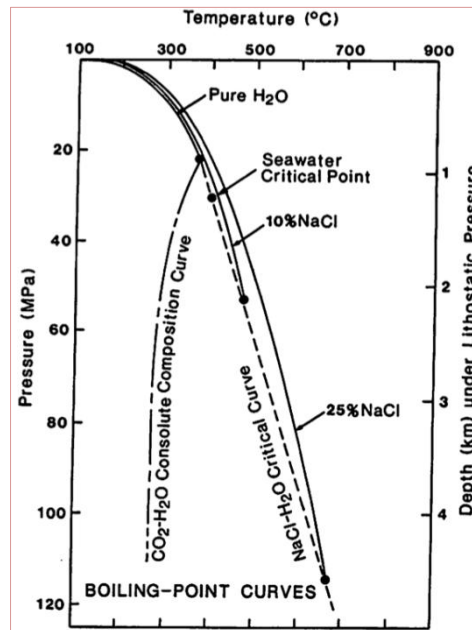
Fig 1.7.6. La figure 7.1 de Formation d'argiles dans des milieux hydrothermaux, par A Inoue, montre les points critiques de l'eau dans un graphique température-pression. L'eau a un point critique à 374 C et 22 MPa.
