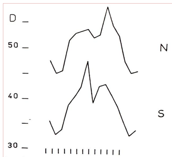
Fig I.10.3. Le libellé de la figure de Piccardi (« Fig 65 ») est : « Variation annuelle de l'essai D dans les hémisphères nord et sud (latitudes moyennes). Sur l'abscisse : les douze mois de l'année. Sur l'ordonnée : test D. Moyennes mensuelles de deux ans. Les minima d'hiver et d'août apparaissent ensemble dans les deux hémisphères. Ils ne dépendent pas d'un effet saisonnier : l'été thermique au nord et l'hiver thermique au sud et vice versa, de Piccardi, 1962. »
