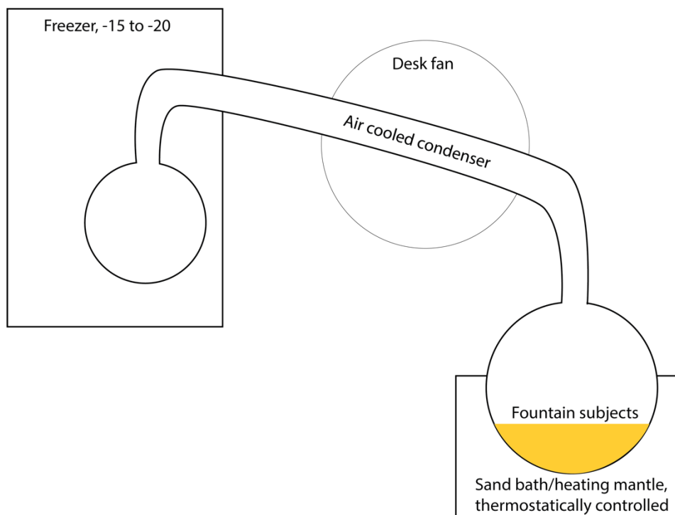
Fig III.4.6. Schéma d'un appareil de fontaine DMSO. Évacuation de la pression non représentée. Cet appareil est également utile pour les systèmes autres que les systèmes basés sur le DMSO, comme indiqué précédemment dans le chapitre.
