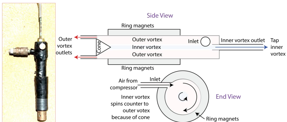
Fig 1.9.3. Le double piège à air vortex. Il s'agit d'un appareil de vortex constitué de tubes en laiton et d'un cône en laiton. Hyper-Air est concentré dans le flux d'air du vortex intérieur. Le vortex de gaz intérieur refroidi est tassé et fait des bulles dans un milieu liquide tel que l'eau ou tout autre liquide. Le gaz chaud est éjecté du vortex extérieur.
