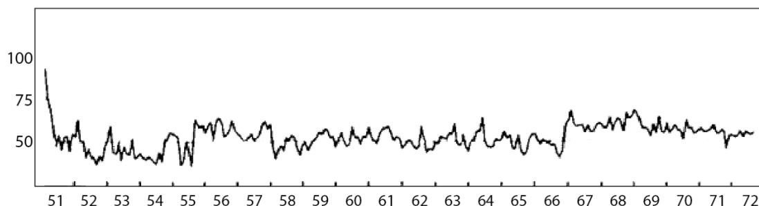
Fig 1.10.2. Piccardi F Test, moyennes mensuelles. Il montre les fluctuations dans le temps du taux de sédimentation de l'oxychlorure de bismuth hydrolysé, de Piccardi, 1962
