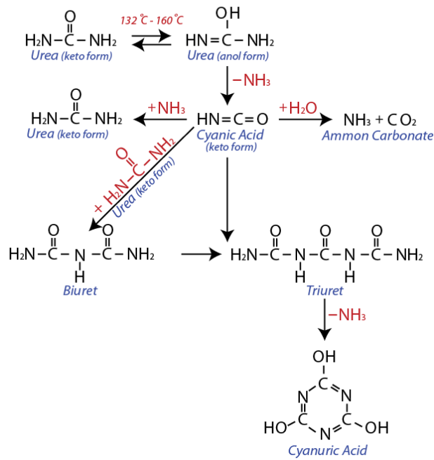
Fig III.1.3. Formation de biuret dans les fondus d'urée. Les voies chimiques mettent en évidence la nécessité d'éliminer l'ammoniac pour maximiser la production de biuret à partir de l'urée. Reproduit de Redemann, 1958. La température de la fonte est importante et si elle est supérieure à 180 C, la fonte produira du triuret.
